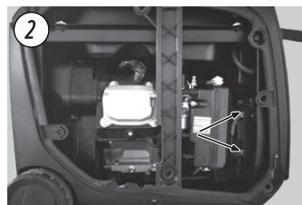
2. Připojte svorky dle správné polarizace („+“ na „+“, „-“ na „-“).
