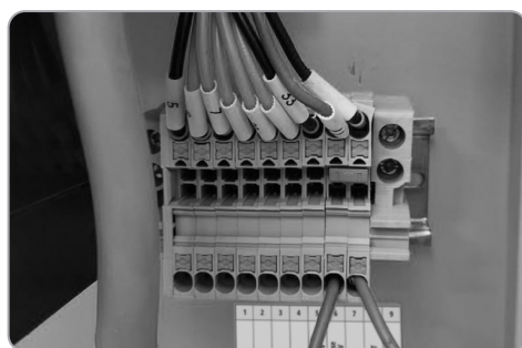
Contacts de commande pour fonctionnement externe
